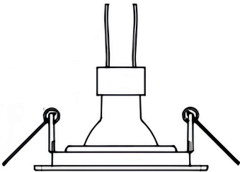
VISTA LATERAL
