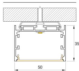
DESENHO TÉCNICO - SLED 9021SF K50
