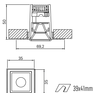
SUPORE PARA FIXAÇÃO NO FRAME
