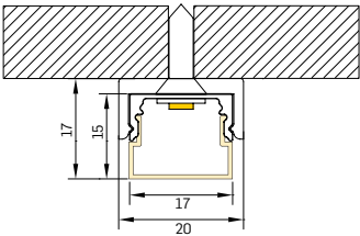
DESENHO TÉCNICO SLED 9005U
